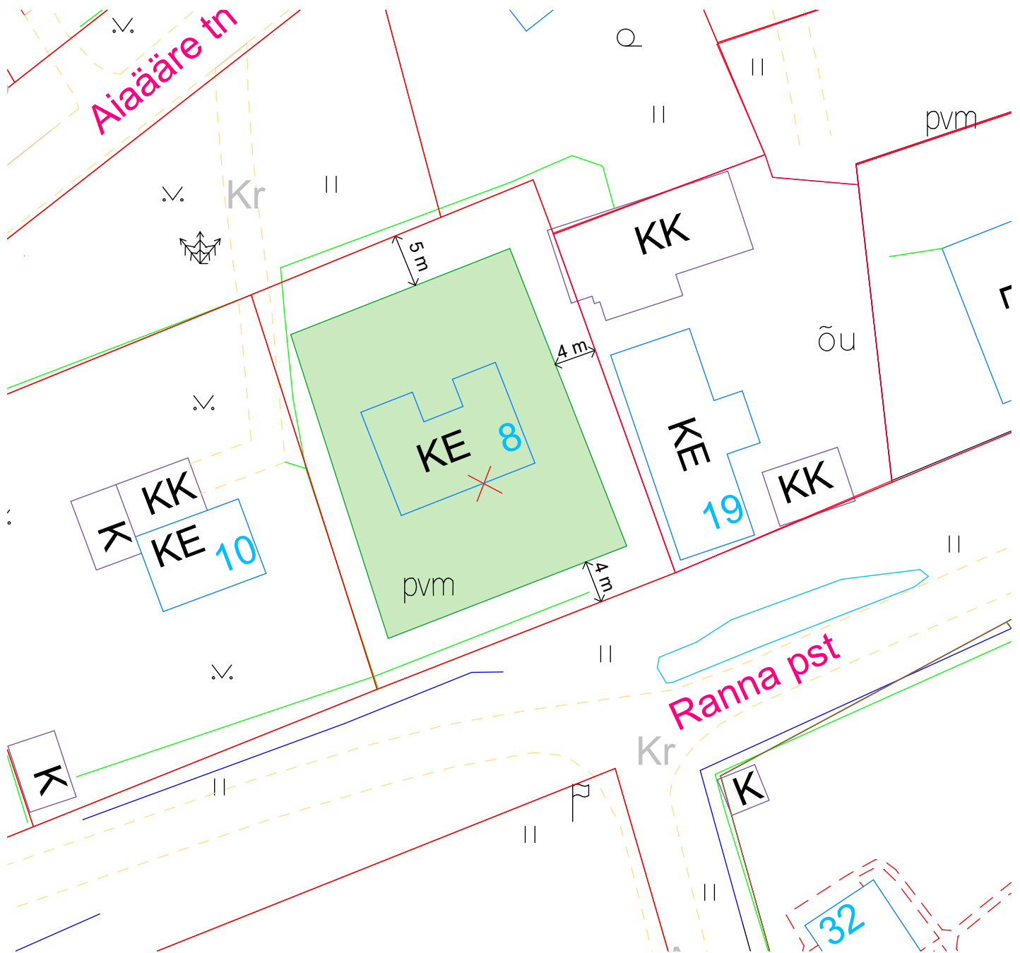
Lisa. Aiaääre 8 ehitusala skeem PTH-20-099
